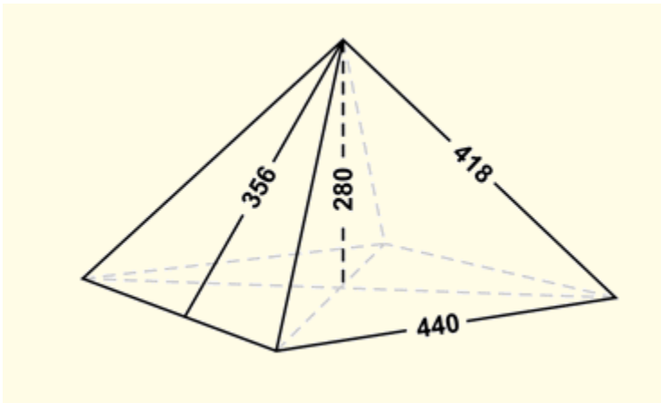
Dimensioni della Grande Piramide in cubiti reali
